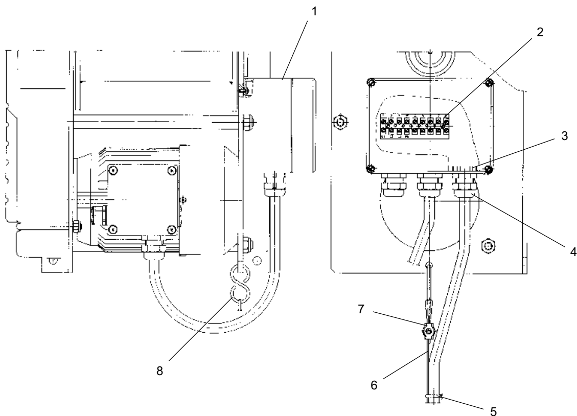
Abb. 14: Direktsteuerung
