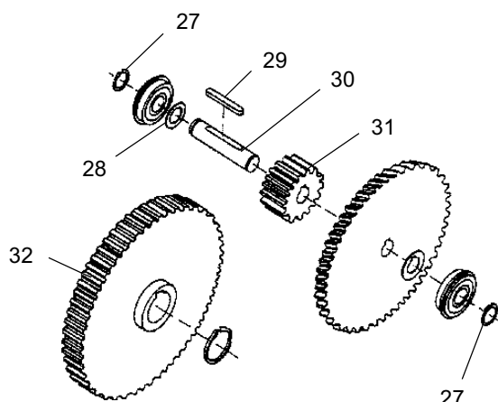
Abb. 12: Getriebeteile für RPE 2-13
