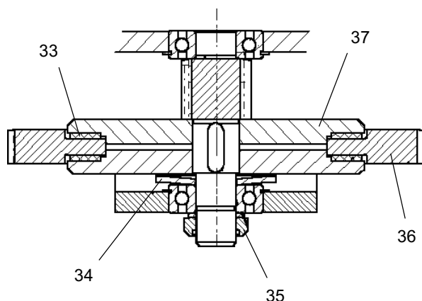
Abb. 13: Rutschkupplung für RPE 10-6
